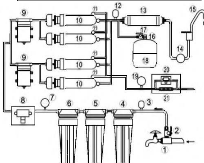
NW-ROC4-400GPD
