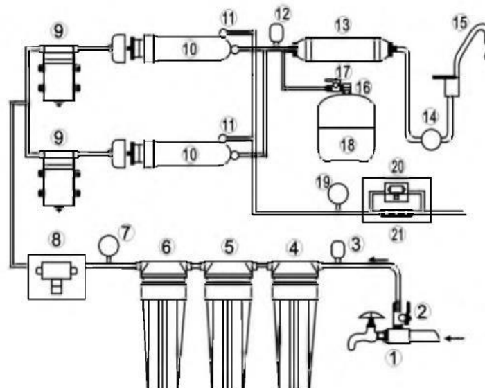
NW-ROC4-200GPD
